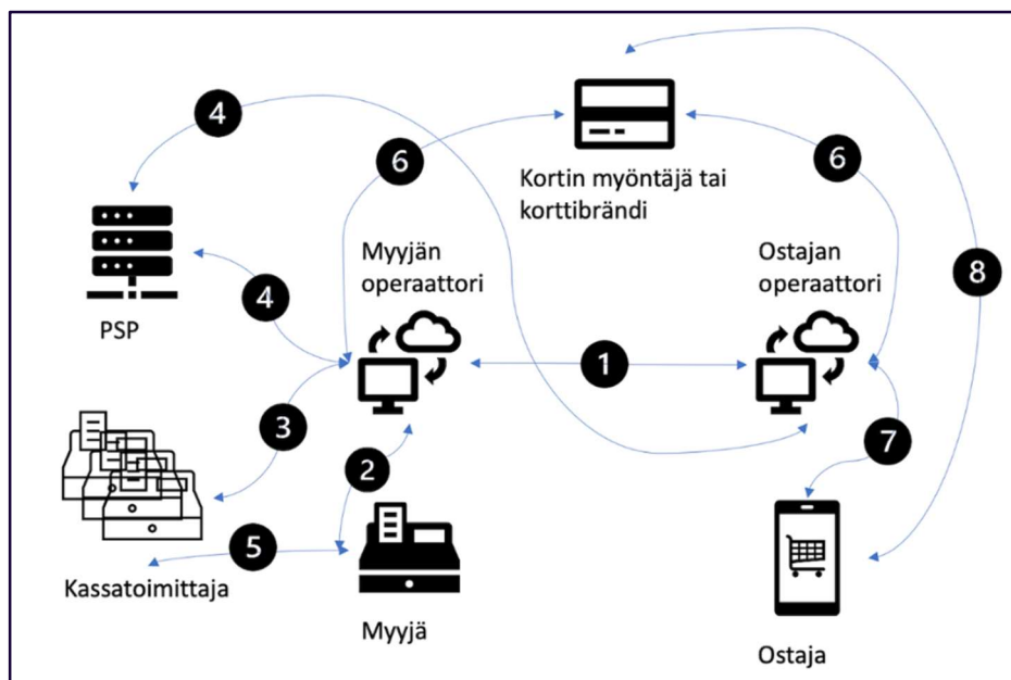
Kuva 3. Nelikulmamallin sopimussuhteet
