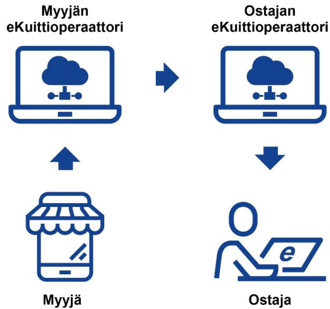
Kuva 1. Nelikulmamalli
